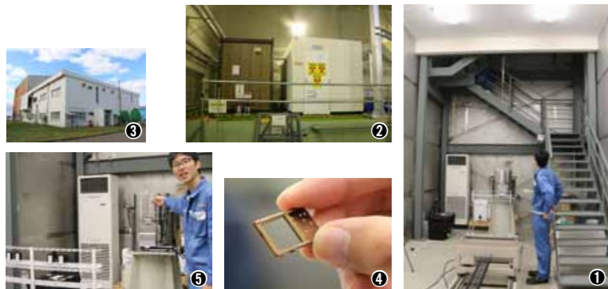
①地下6mにある放射線照射施設。中央奥の円筒の装置から放射線がビームのように出るといふ。②照射施設の入り口。「管理区域」というマークに少し緊張する。③施設はAMSが設置される大きな建物の前にある。④これが積算線量計。正方形のガラスのような面を放射線がどのくらい通過したかを測定する。⑤線量計を写真左下のように並べ、放射線を照射する。⑥敷地の外にある百葉箱。ここでも積算線量計は放射線を計測していた。
