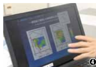
①六ヶ所村再処理工場沖合約3kmに設置される係留式ブイ。海水の流速流向、水温、塩分などの観測データが大湊の研究所に送られてくる。②左が流向流速計で、右が水中放射線センサー。係留式ブイの下に装着される。③こちらが送られてきたデータを観られるシステム。このデータを用いてシミュレーションモデルを作っていく。④シミュレーションモデルの画像。六ヶ所村周辺海域の海の動きがわかる。
