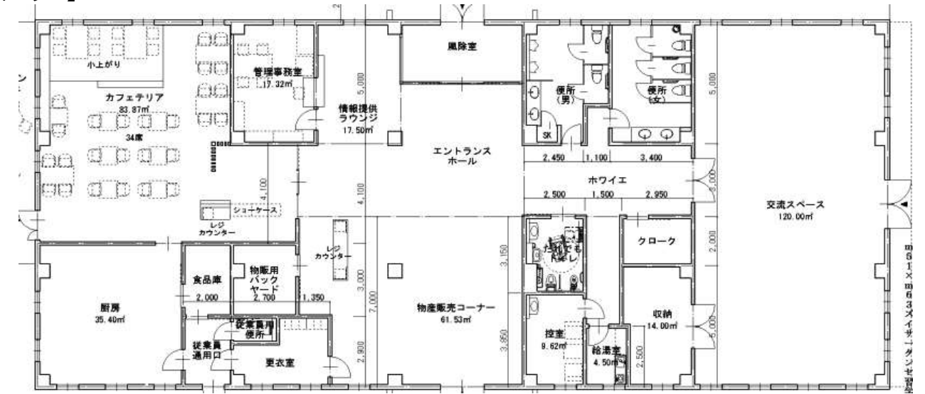
【平面プラン】
